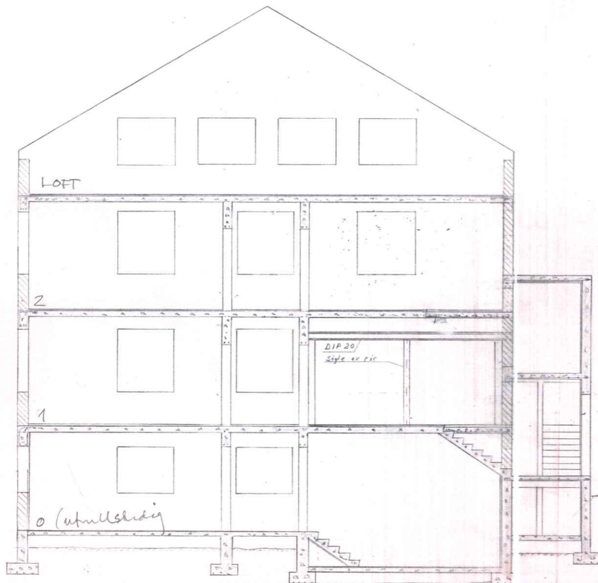
snitt A-A
